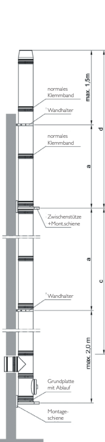
ICS Ø80-300
