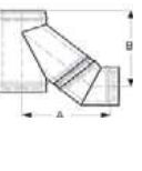
Abb. Rauchrohranschluss 45° mit Bogen 45°
