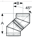
Abb. Bogen 85°
