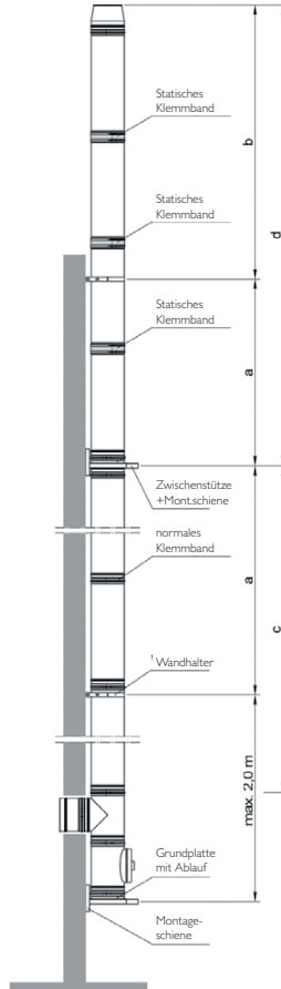
ICS Ø80-300
