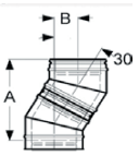
Abb. Bogen 45°
