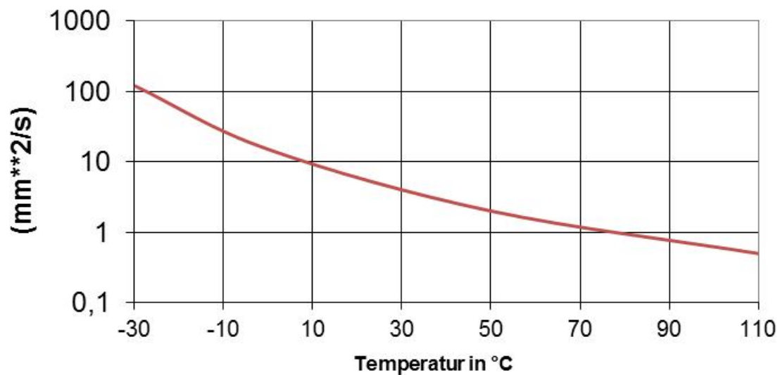
Viskosität ( mm 2 /s ) Solarliquid L gebrauchsfertig
