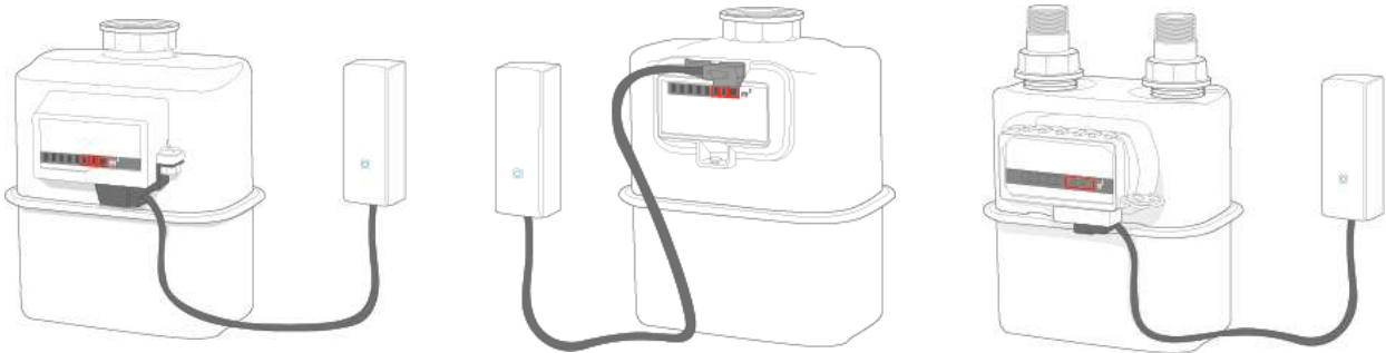
Abbildung 13: Gaszähler-Varianten
