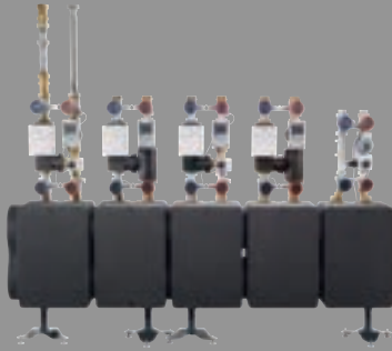
Logaflo HS40 / HS50 HKV2 / HKV3 für zwei und drei Heizkreise
