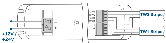
Anschluss RGB Stripe
